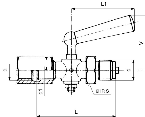
Присоединительные и строительные размеры
