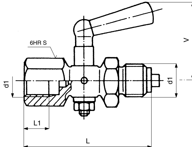
Присоединительные и строительные размеры
