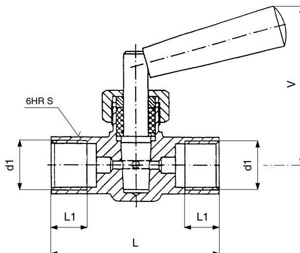
Присоединительные и строительные размеры
