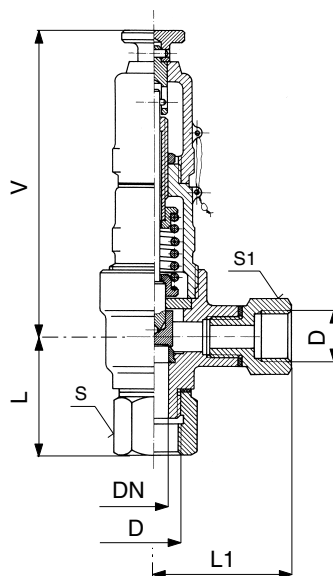
Присоединительные и строительные размеры
